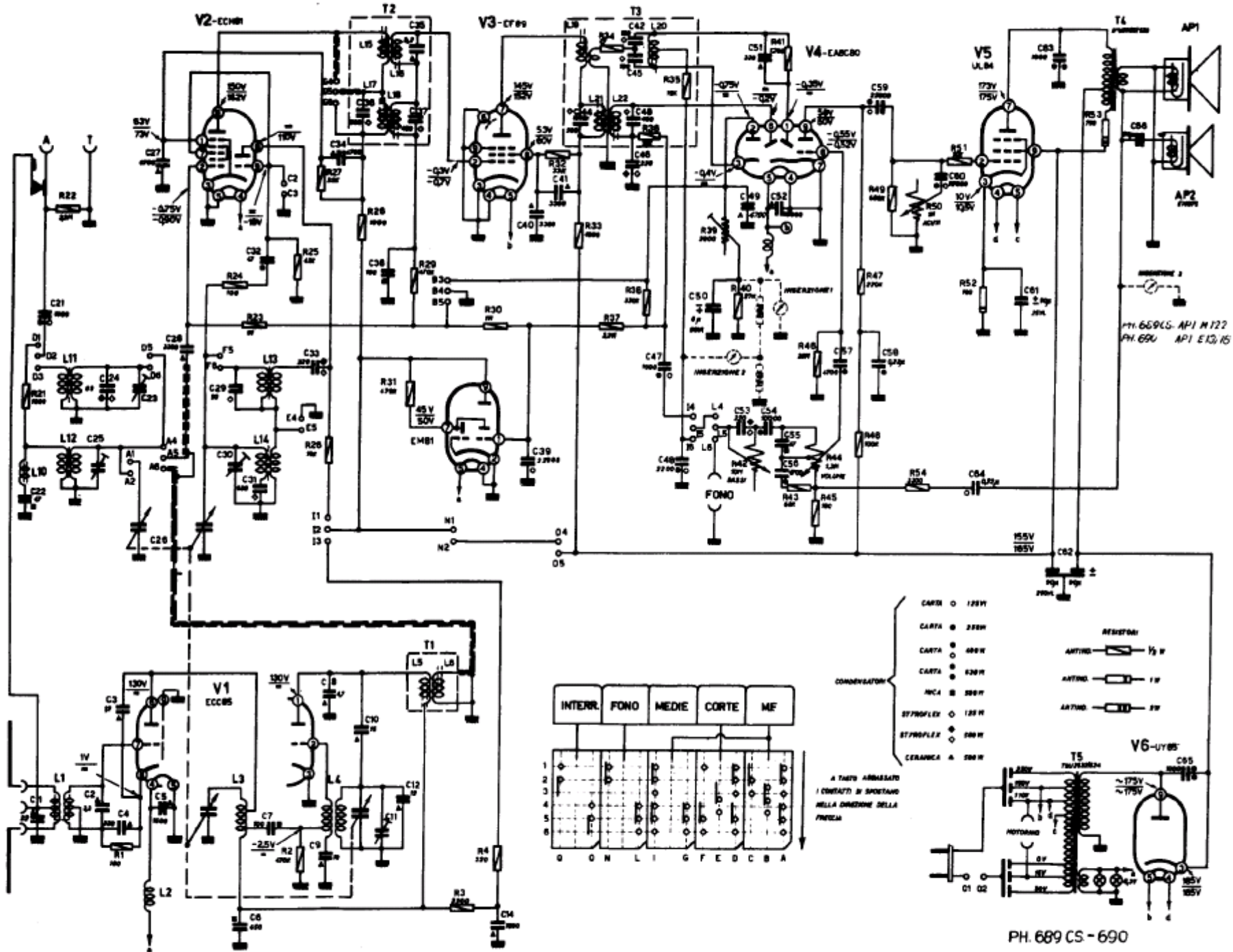
PHONOLA - Modd. 689 e 690. Apparecchio a modulazione di ampiezza e di frequenza, con ricezione della gamma onde medie, gamma onde corte e banda onde ultracorte. Commutazione a tastiera, occhio magico e due altoparlanti. Resa d'uscita 4 watt. Consumo 50 watt.
